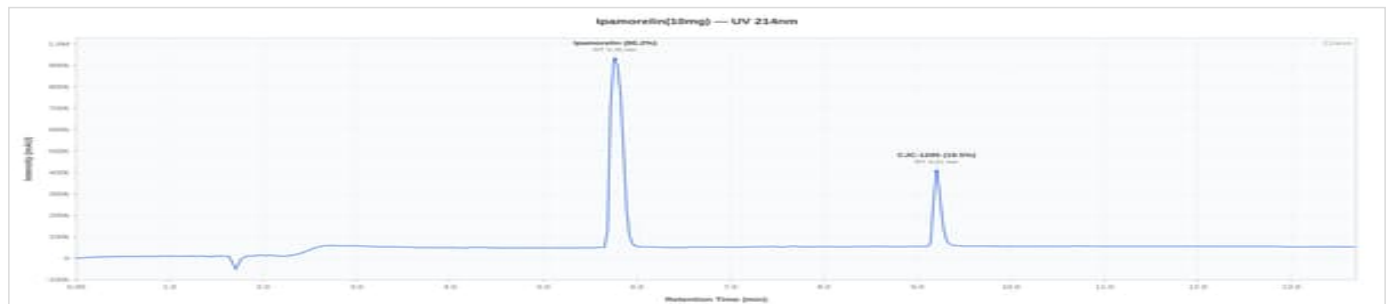
CJC-1295 / Ipamorelin 10mg - QPUSACJCIPA-0021: UV Chromatogram
